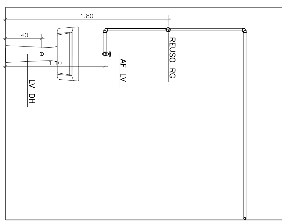
4 Vista 4 ESCALA 1:25
