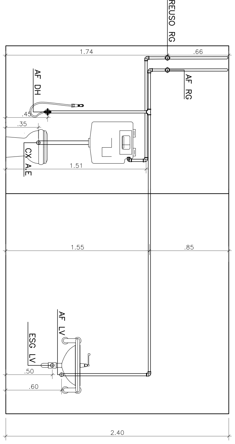
9 Vista 12 e 13 ESCALA 1:25
