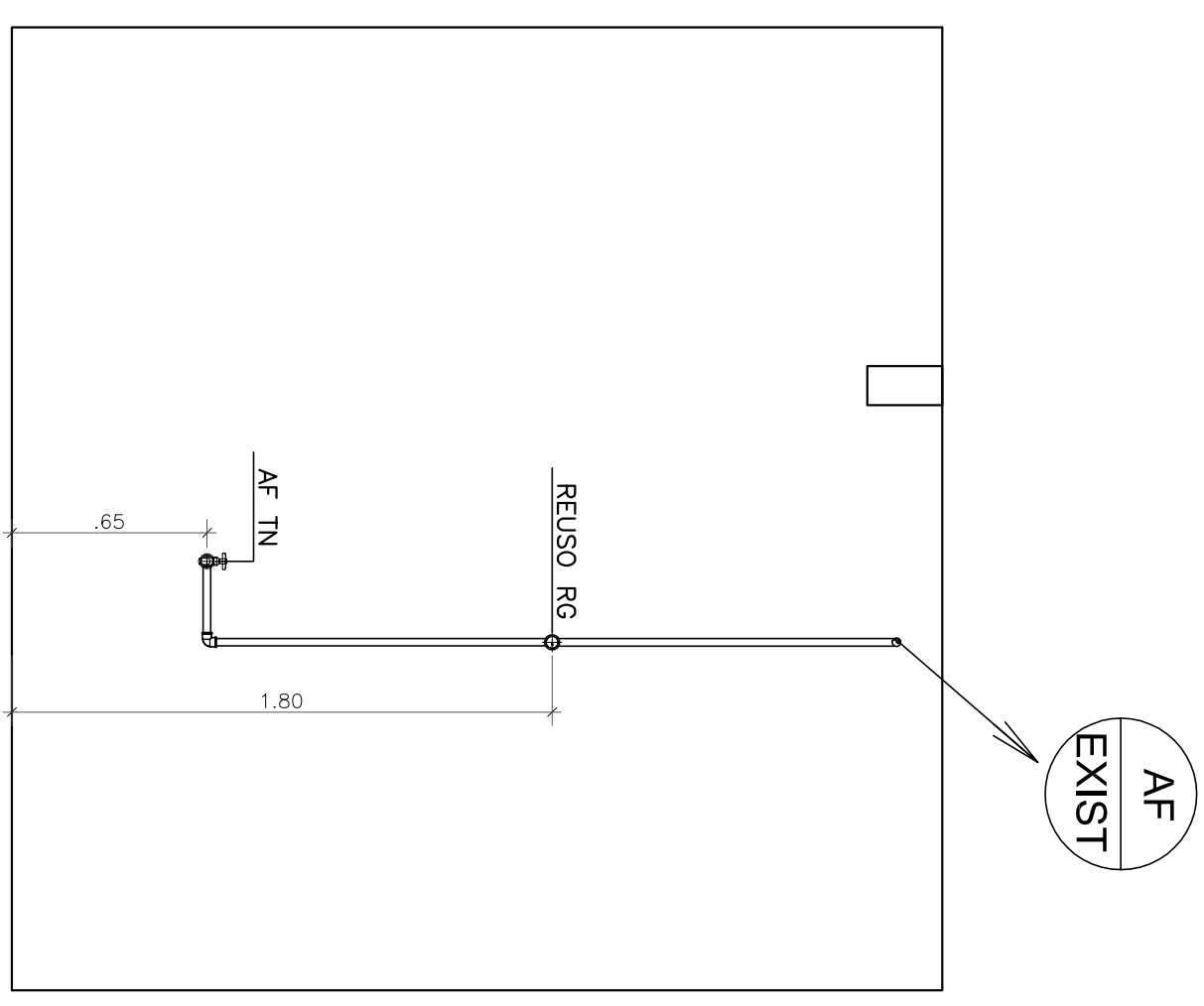
7 Vista 9 ESCALA 1:25
