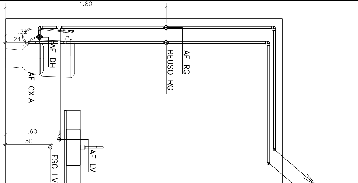
1 Vista 1 ESCALA 1:25
