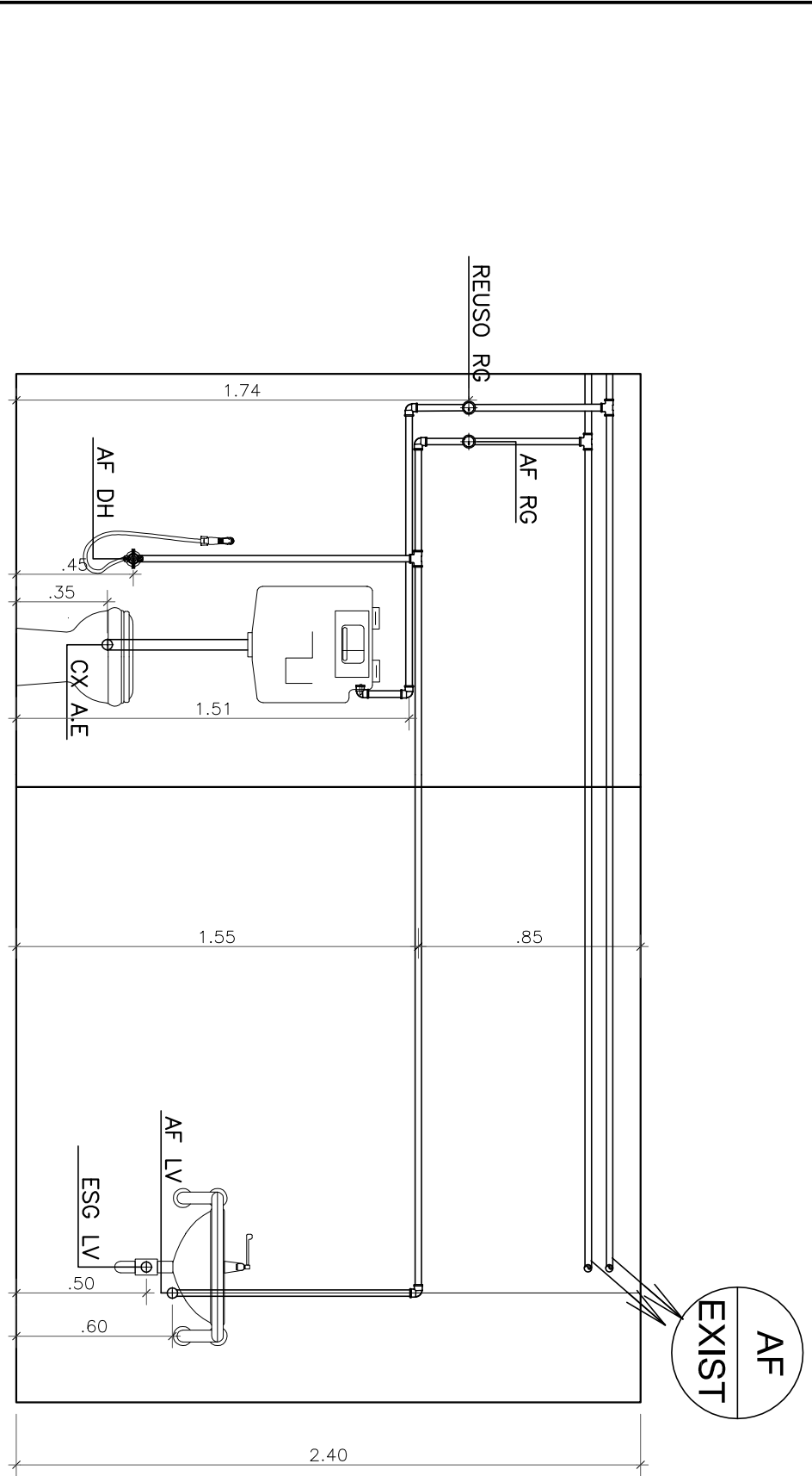
8 Vistas 10 e 11 ESCALA 1:25
