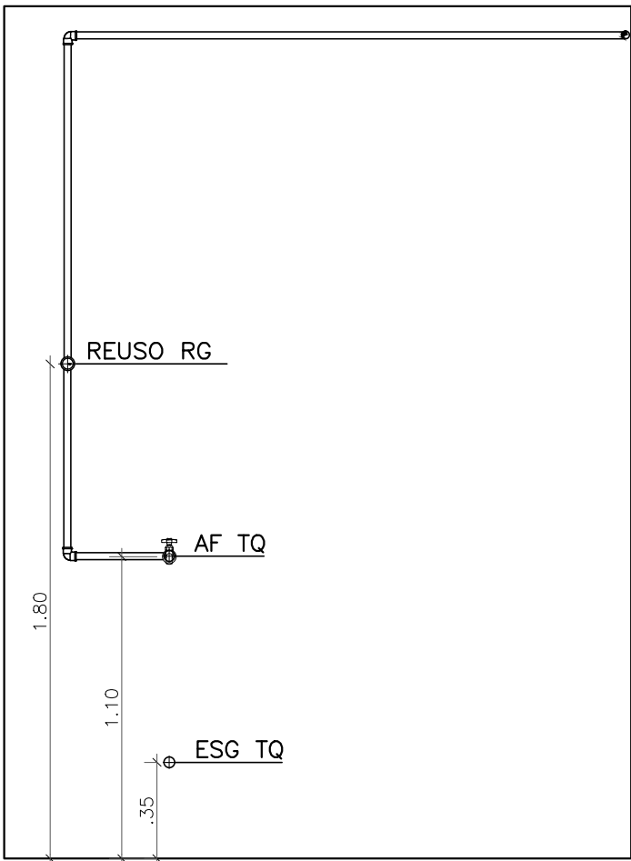
5 Vista 6 ESCALA 1:25
