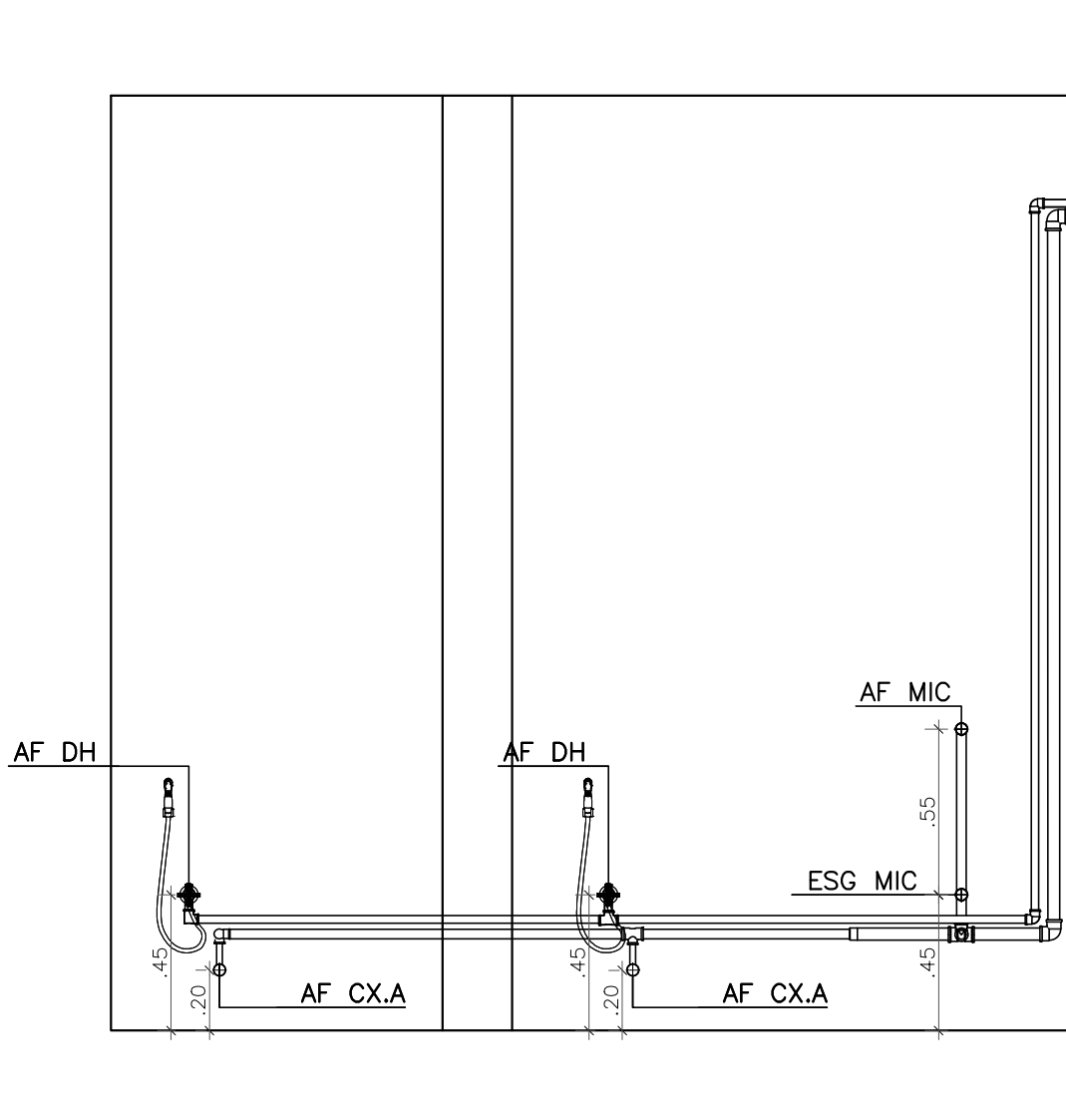
6 Vistas 7 e 8 ESCALA 1:25
