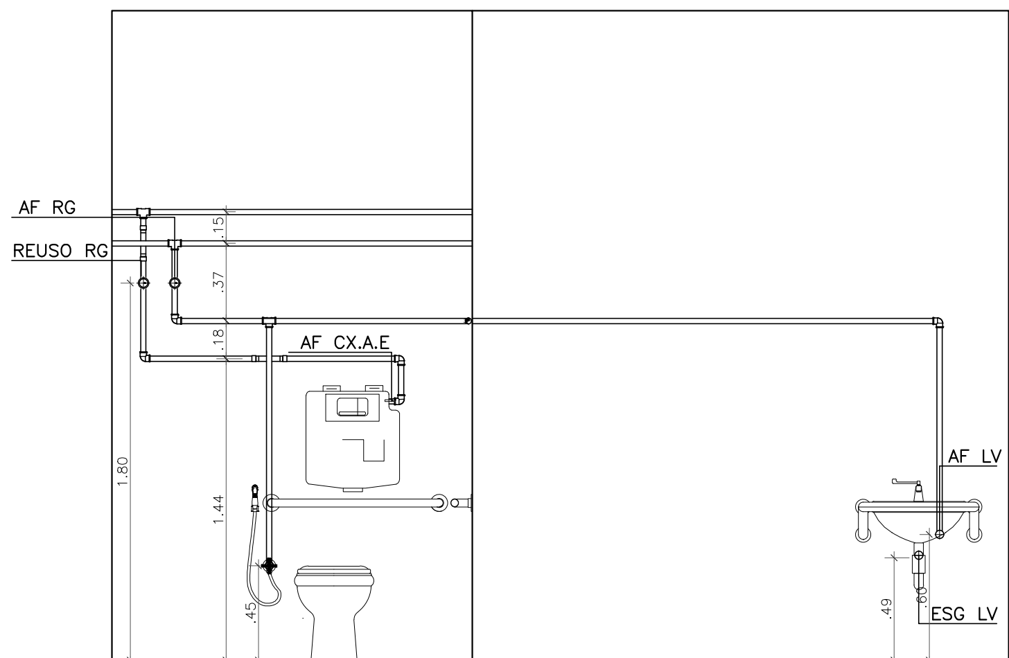
11 Vistas 16 e 17 ESCALA 1:25
