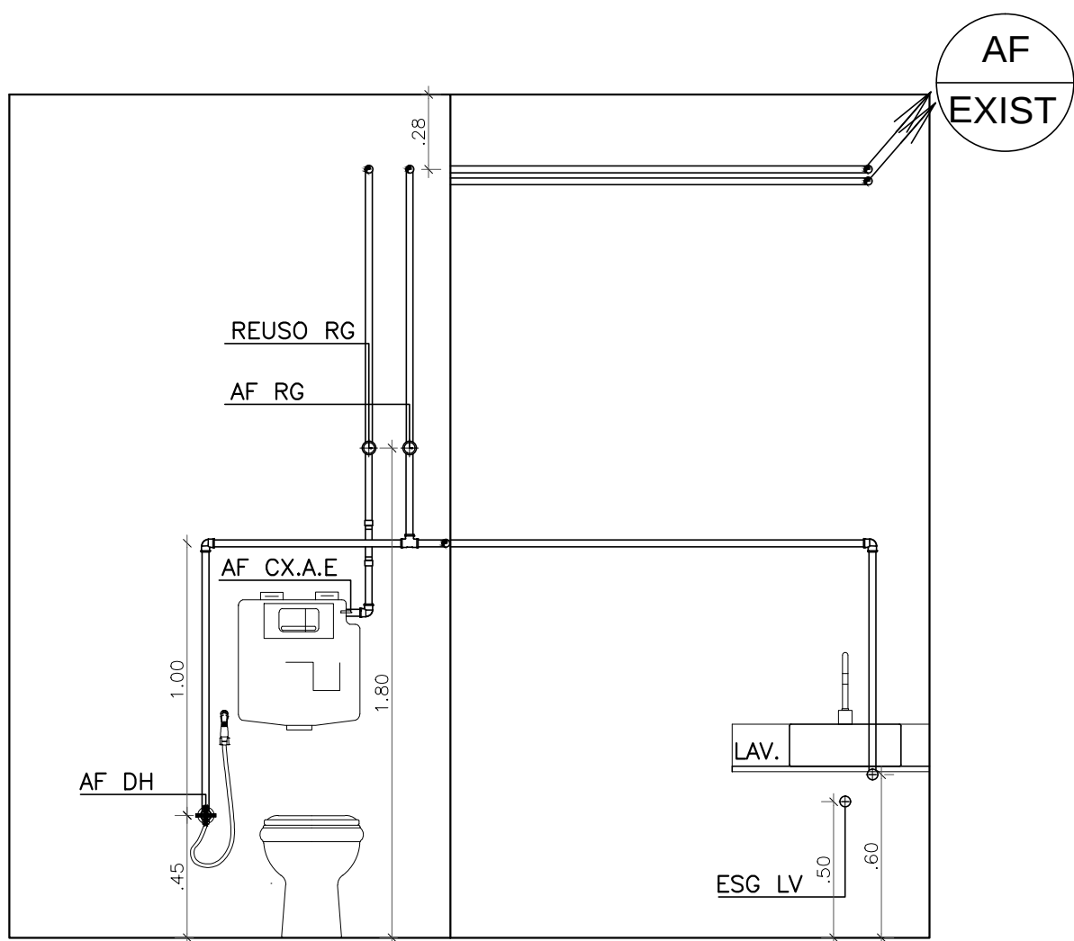
1 Vistas 1 e 2 ESCALA 1:25
