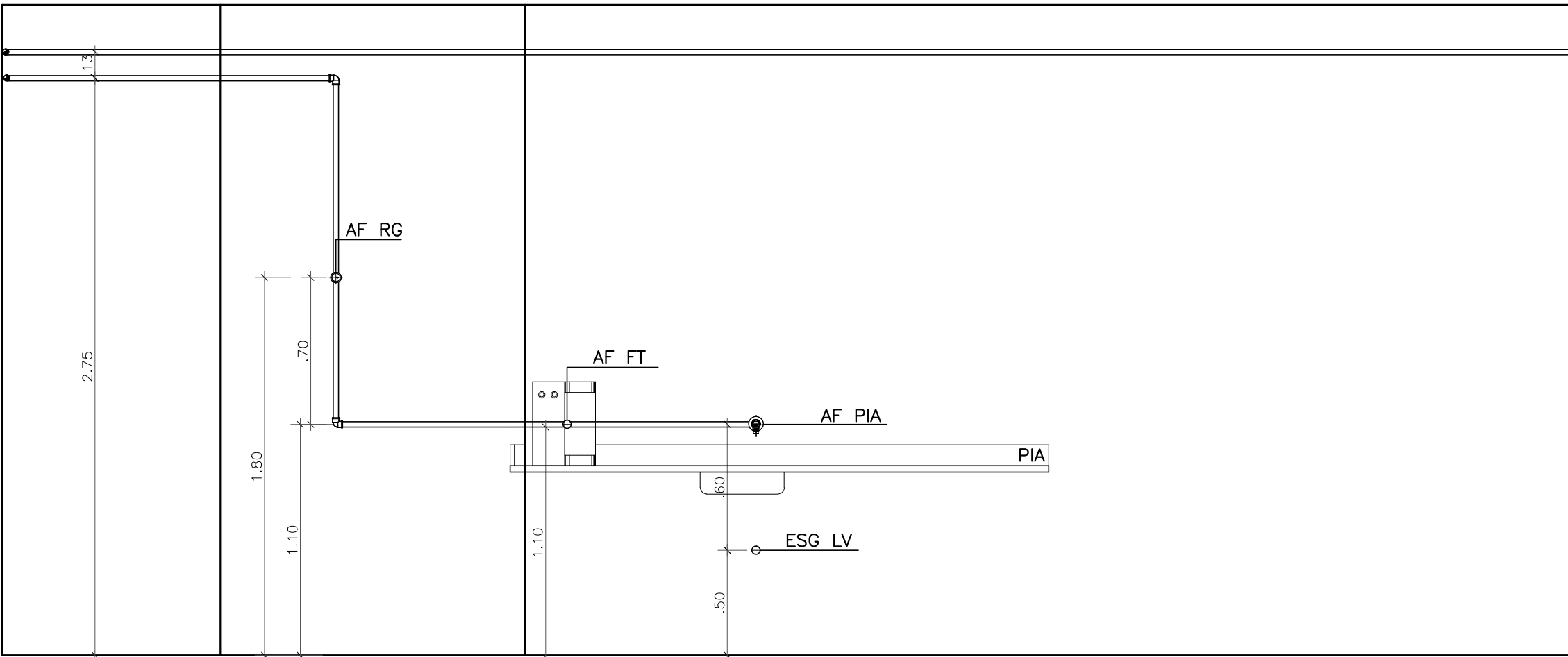
7 Vistas 9 e 10 ESCALA 1:25
