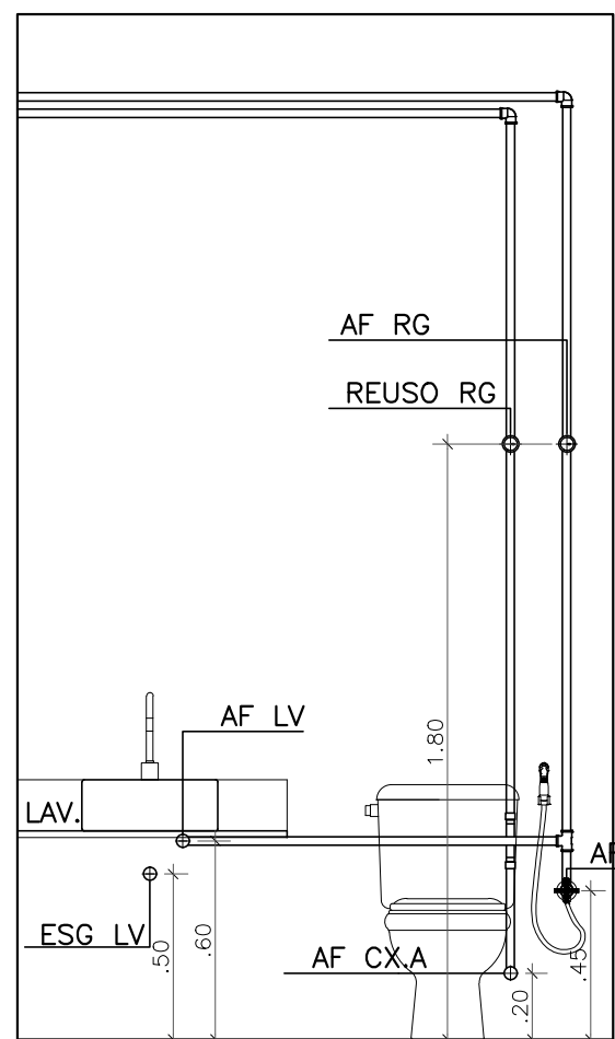
14 Vista 20 ESCALA 1:25
