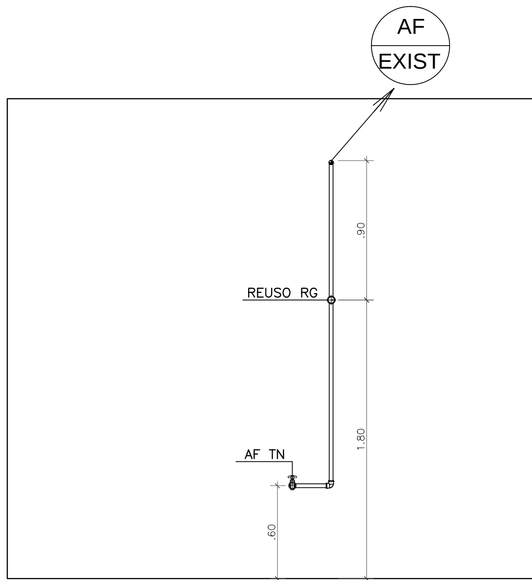
9 Vista 12 ESCALA 1:25
