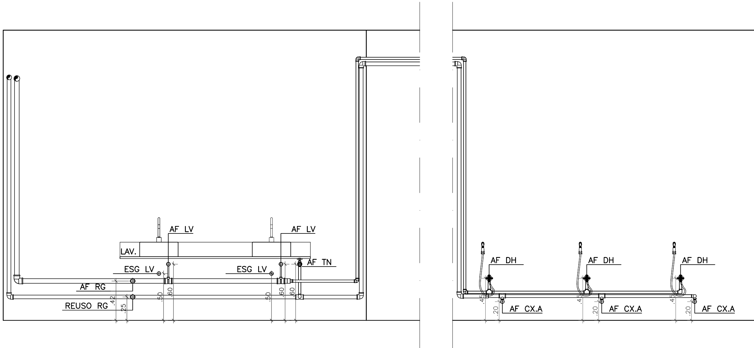
4 Vistas 4 e 5 ESCALA 1:25
