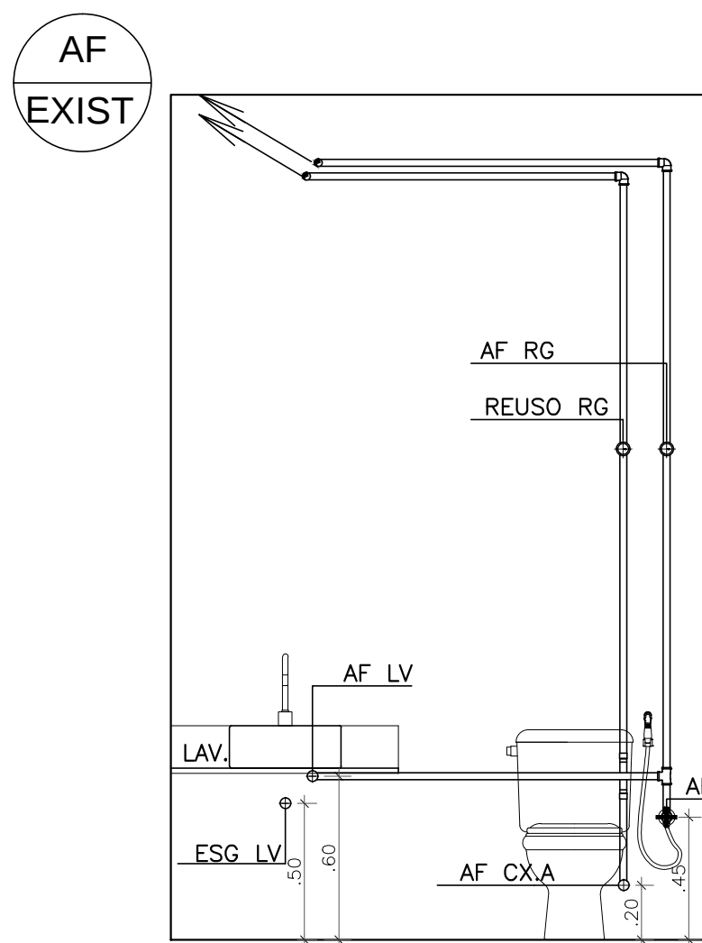
2 Vista 3 ESCALA 1:25
