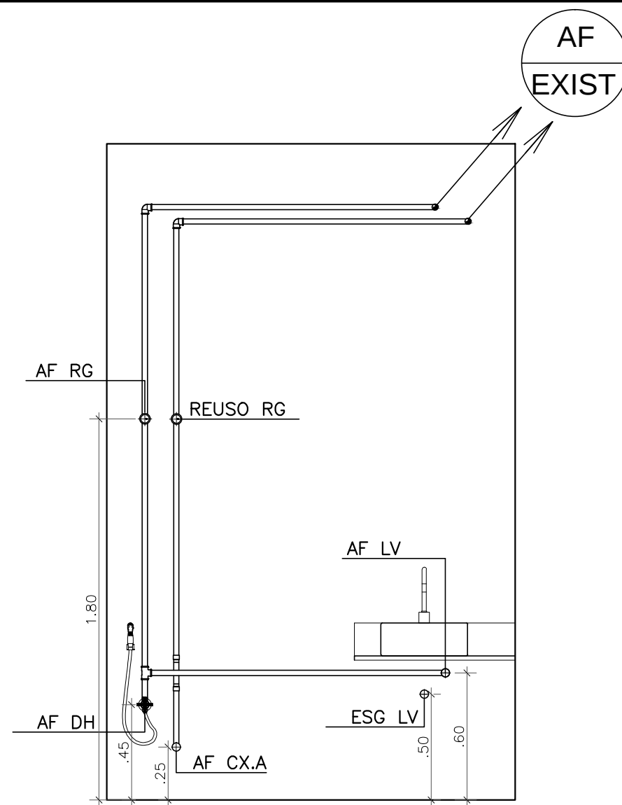
1 Vista 1 ESCALA 1:25
