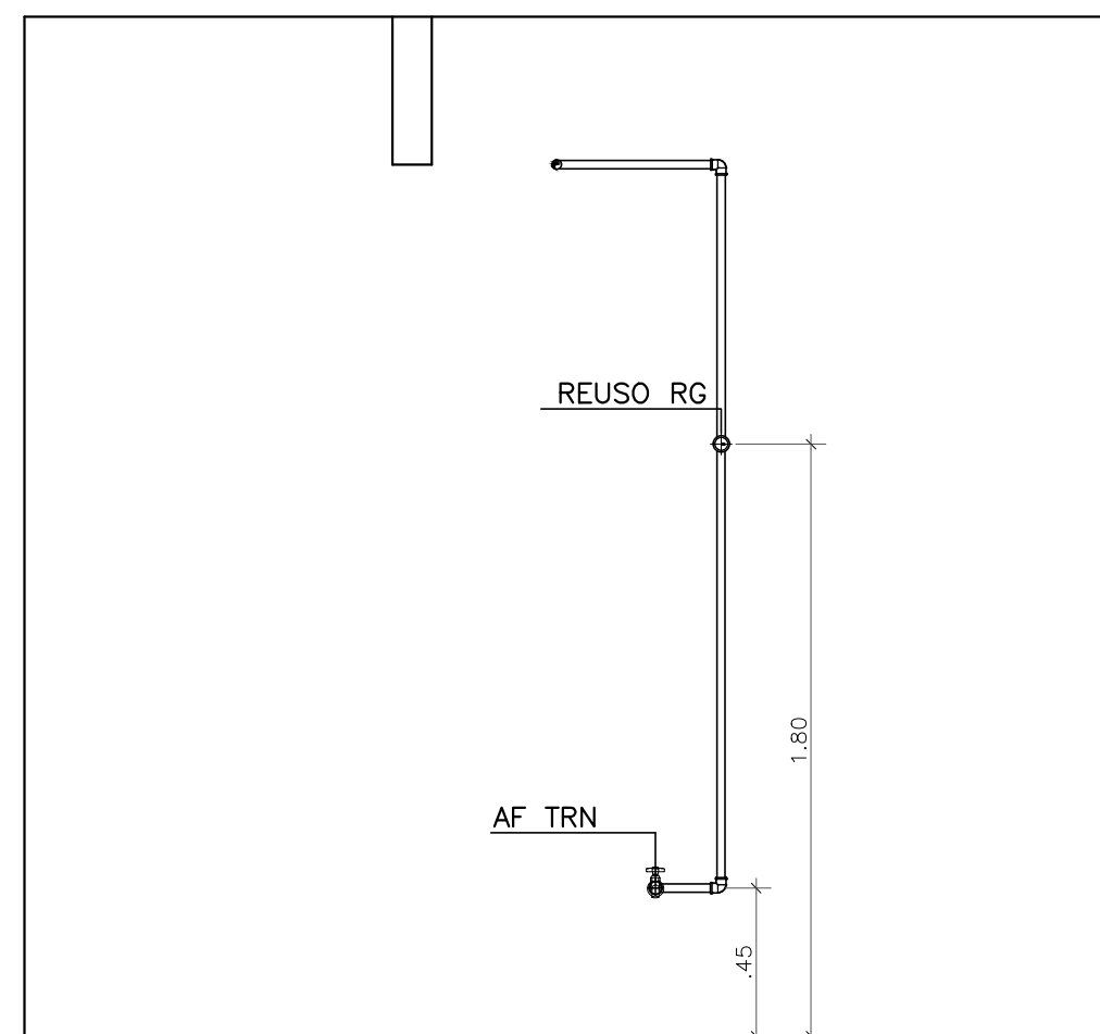
9 Vista 13 ESCALA 1:25
