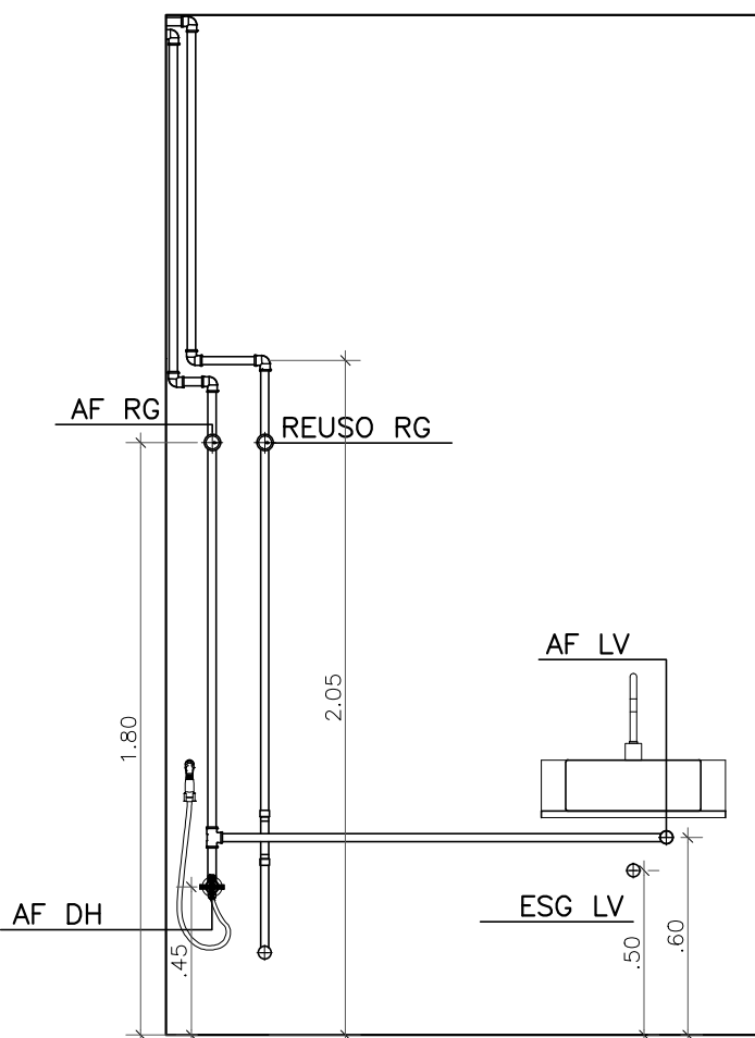
8 Vista 11 ESCALA 1:25
