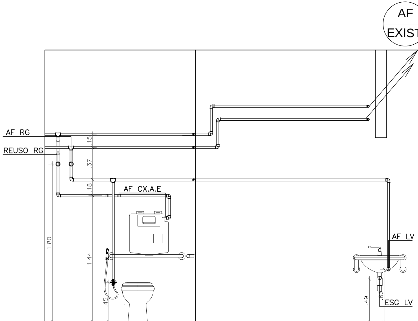
10 Vistas 14 e 15 ESCALA 1:25
