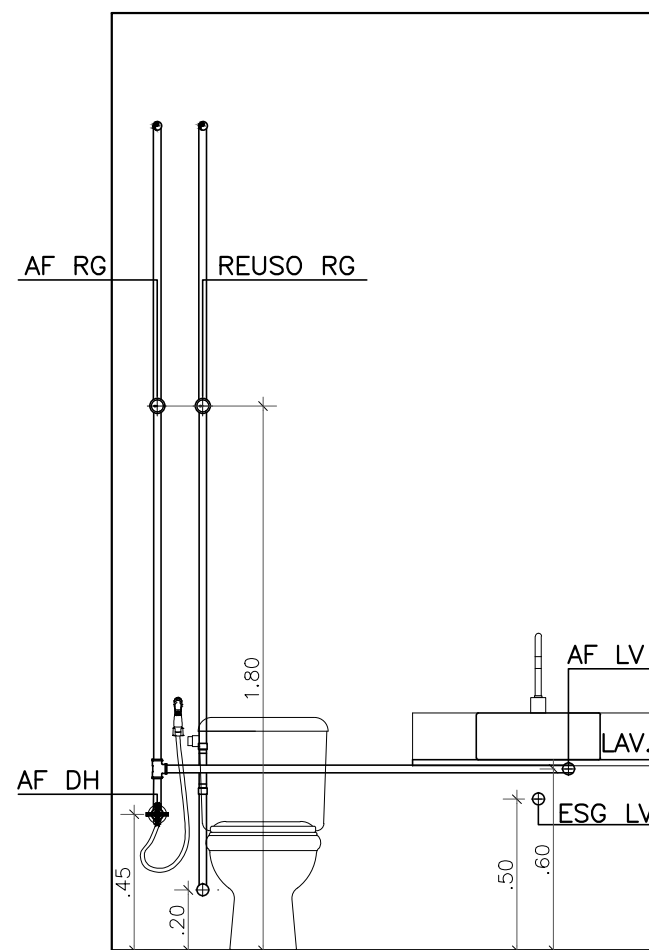
12 Vista 18 ESCALA 1:25
