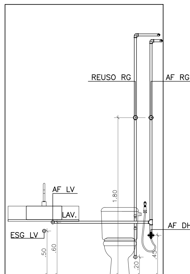
6 Vista 8 ESCALA 1:25
