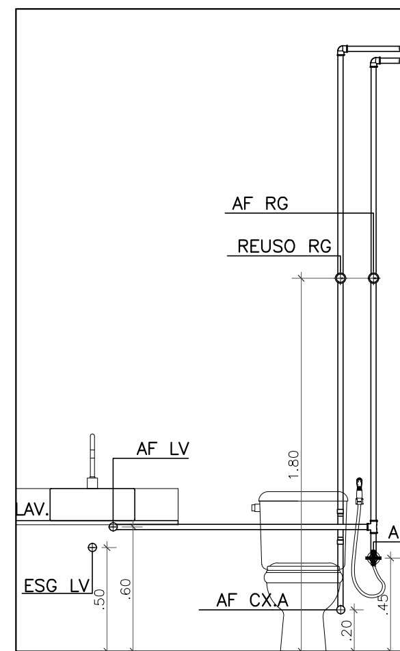
13 Vista 19 ESCALA 1:25
