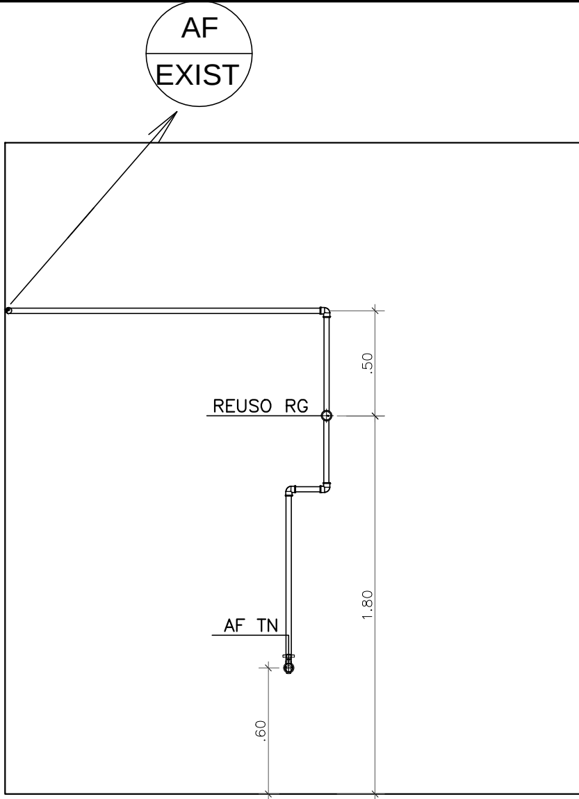
3 Vista 3 ESCALA 1:25
