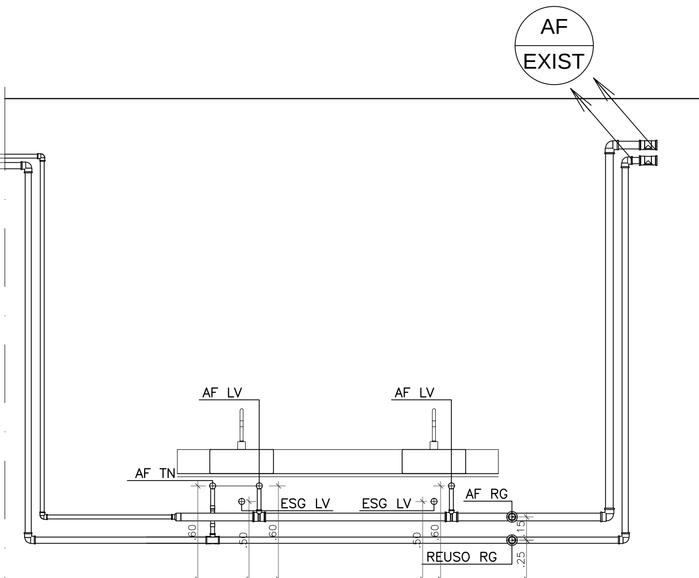
4 Vistas 5 e 6 ESCALA 1:25
