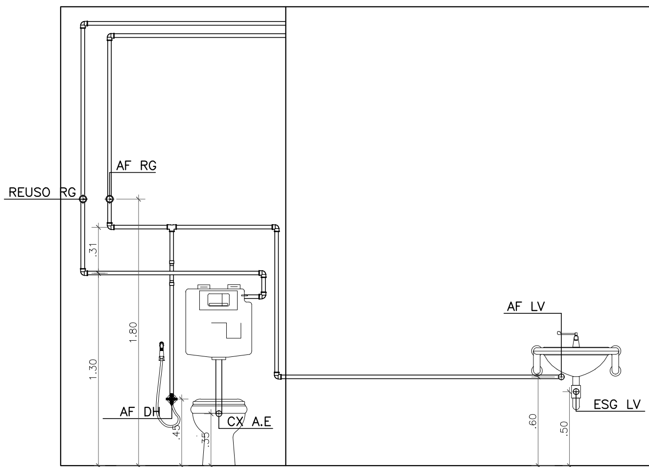
11 Vistas 15 e 16 ESCALA 1:25
