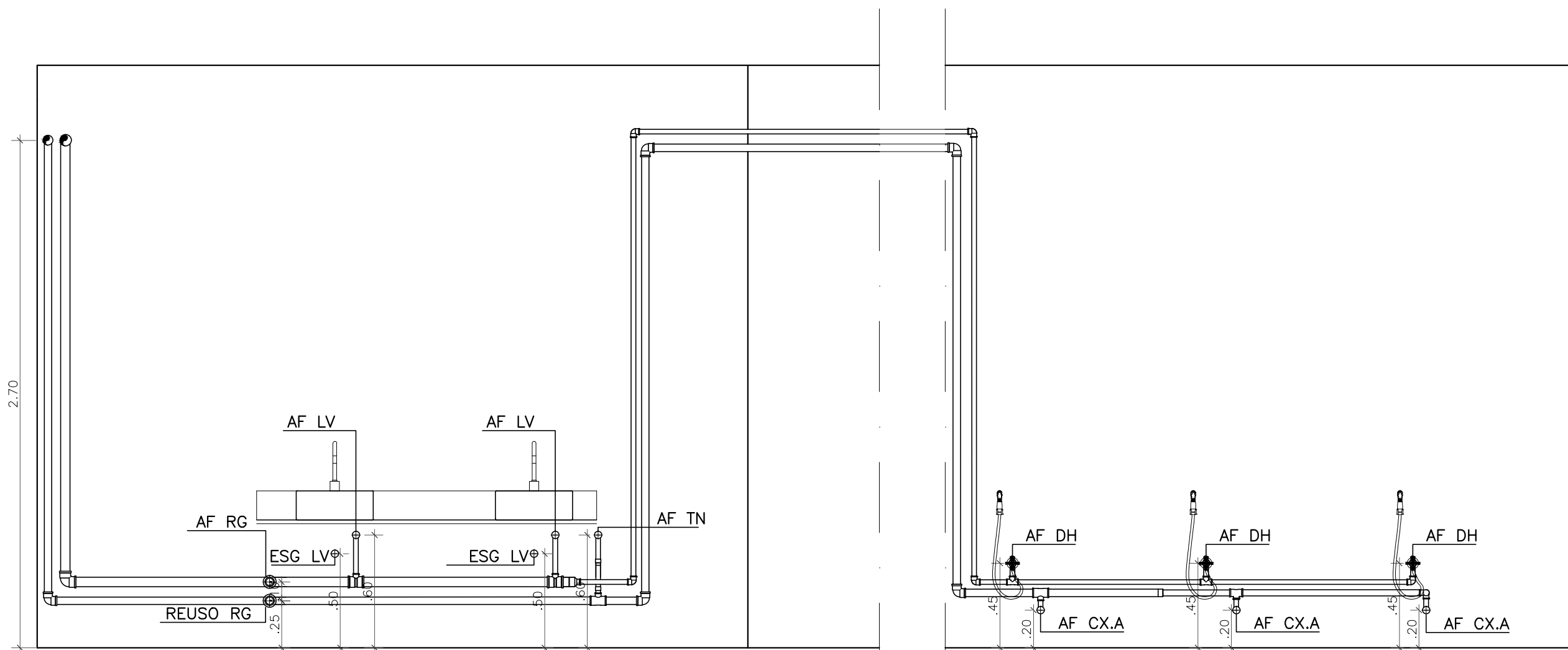
4 Vistas 5 e 6 ESCALA 1:25
