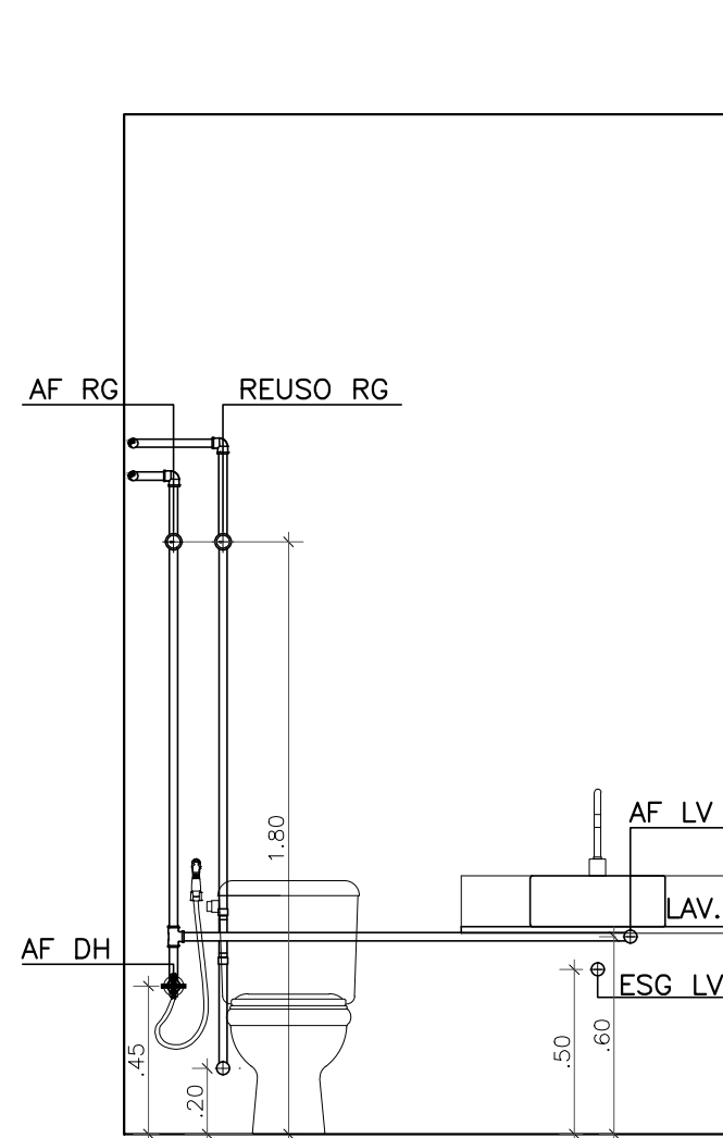
3 Vista 4 ESCALA 1:25
