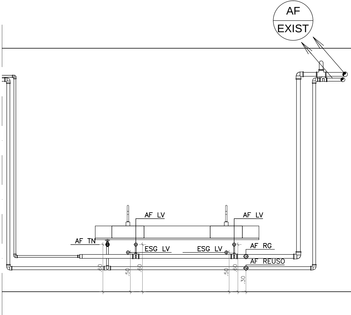
3 Vista 3 ESCALA 1:25
