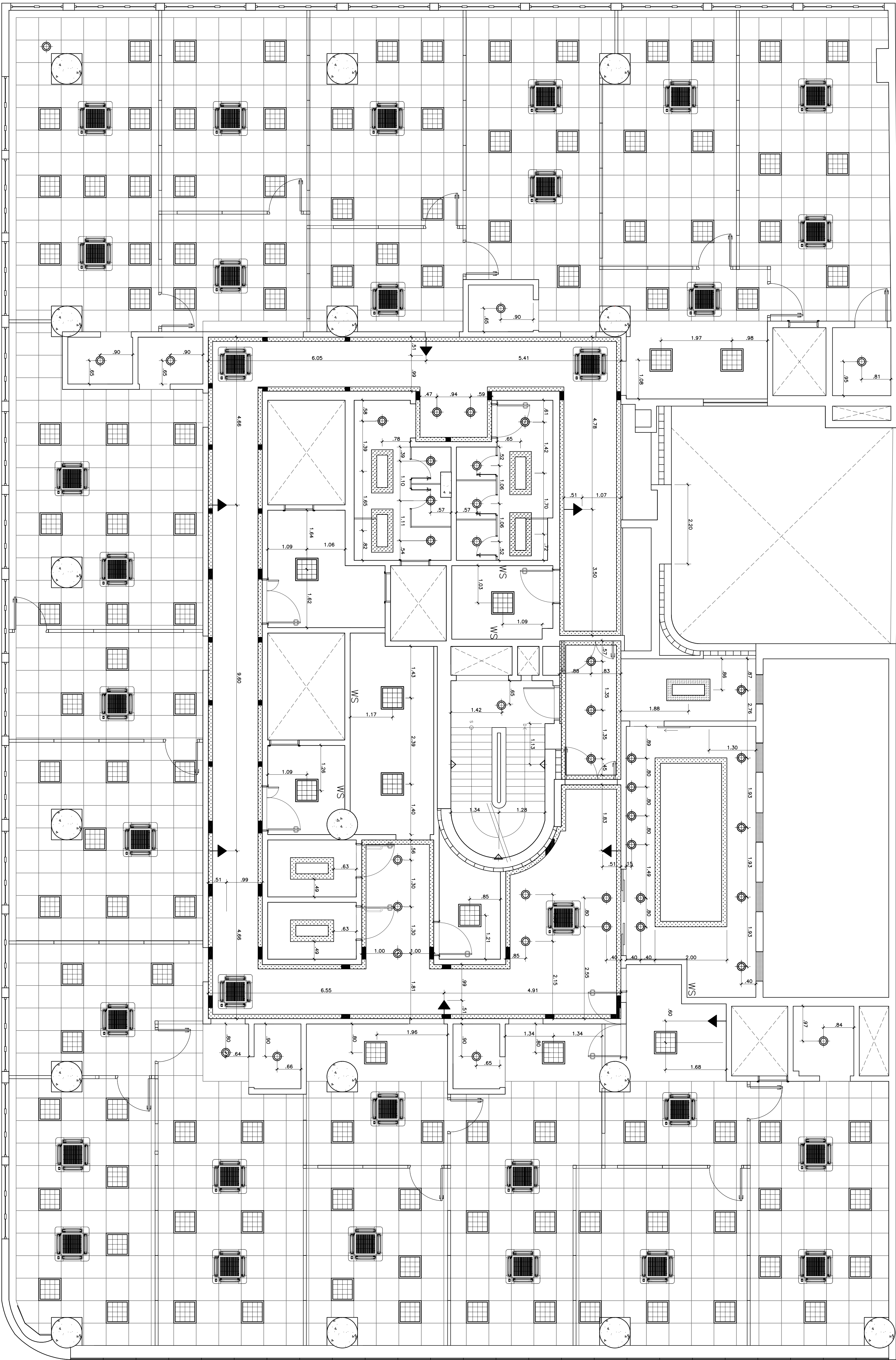
10 AO 16º PAVIMENTO ESCALA 1:50
