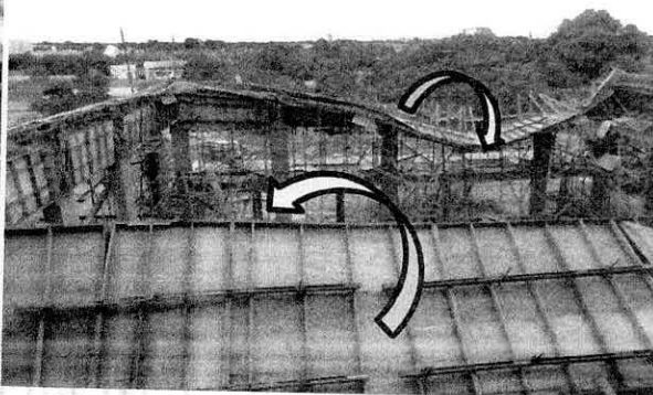
Vetor da parte externa para a interna
