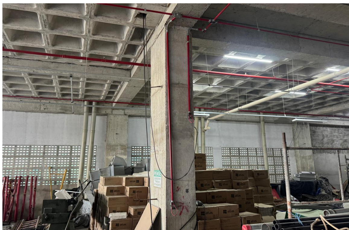
Figura 28. Eletrodutos em aço já com cabos instalados.
