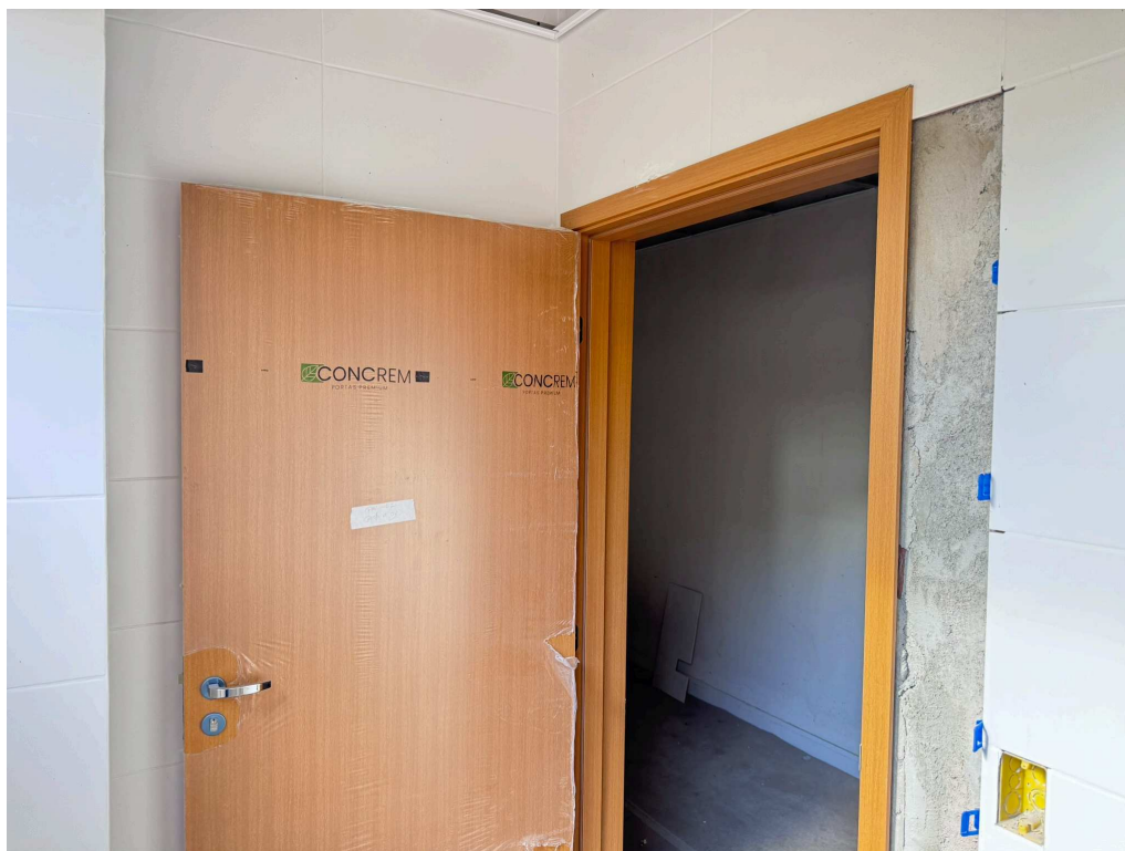
Figura 14 Instalação das portas de giro nos banheiros PCD.
