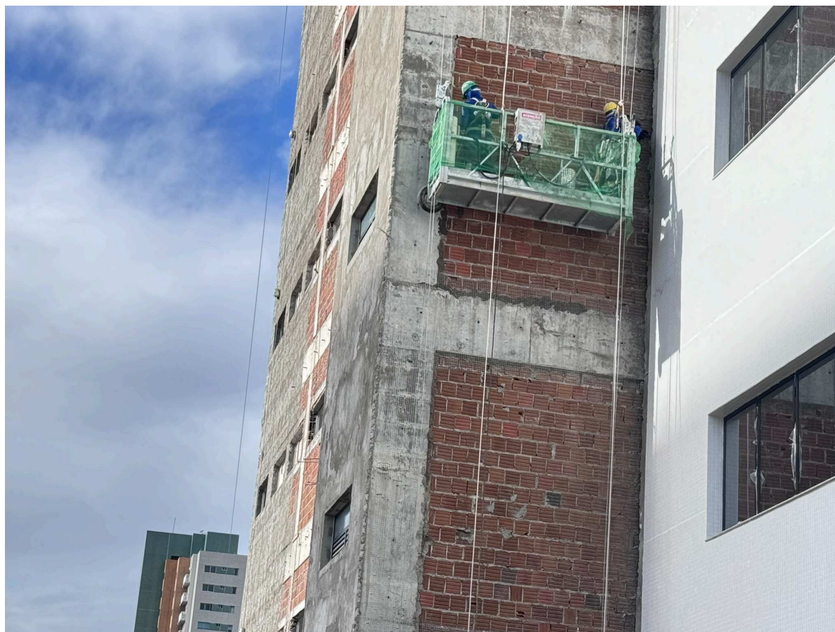
Figura 5 Aplicação de chapisco e reboco na fachada oeste da edificação.
