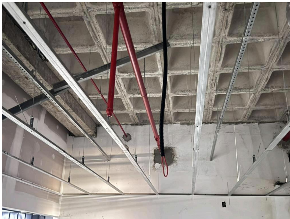
Figura 24 Eletrodutos para sistema de detecção e alarme de incêndio.
