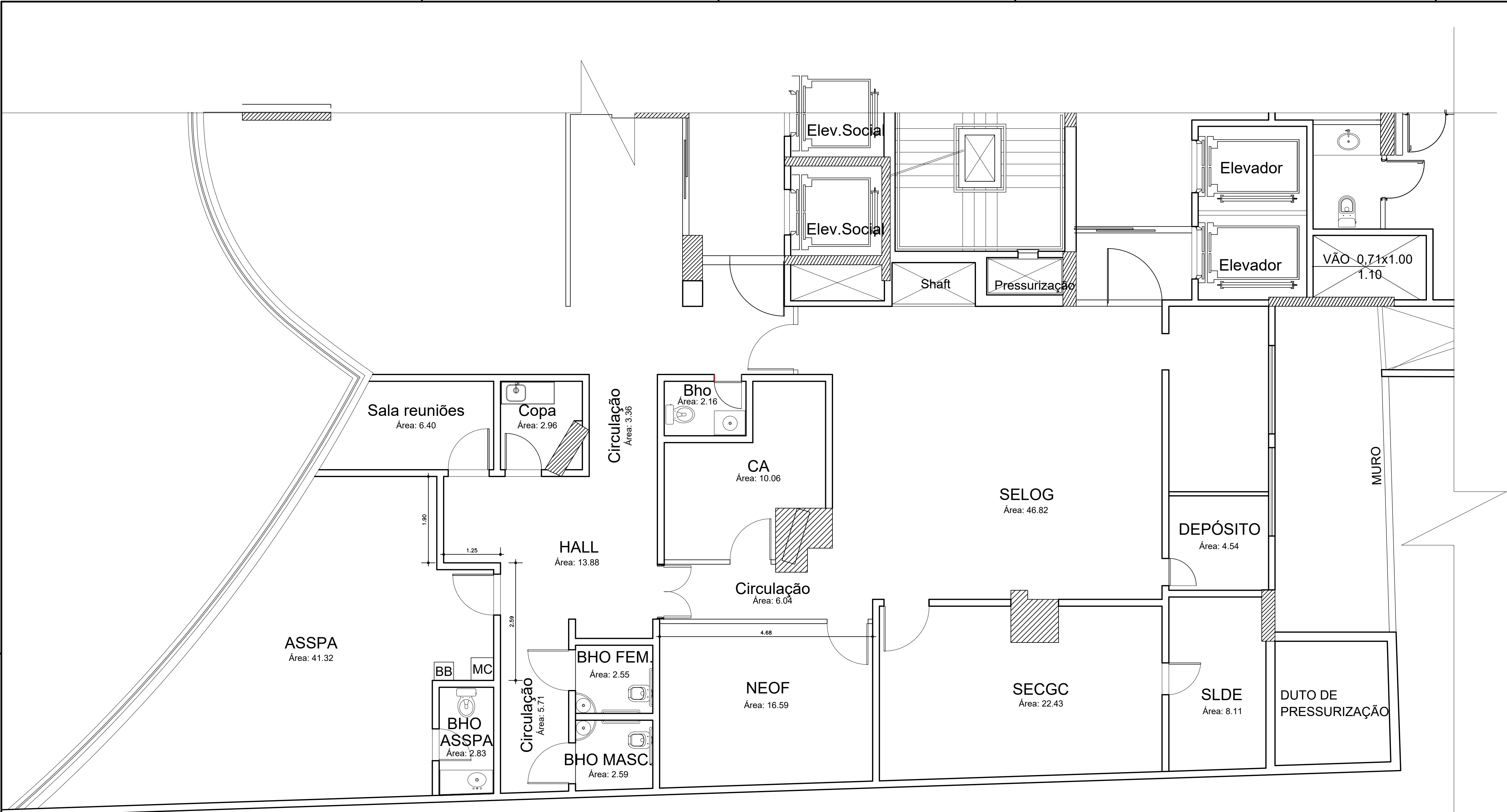
PLANTA BAIXA – 2º PAV. MPF; ED. EVOLUTION escala.....1:50
