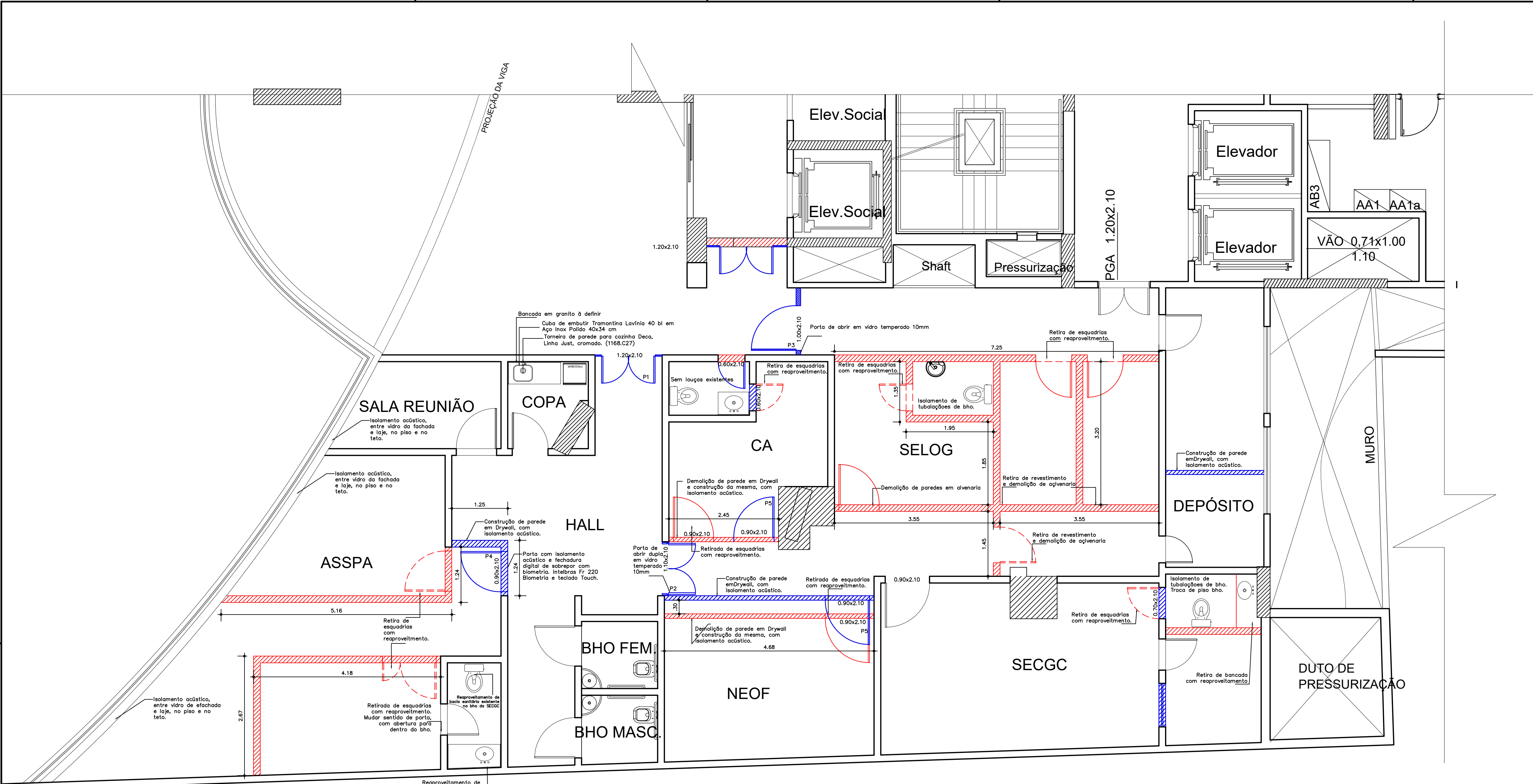
PLANTA DE DEMOLIÇÃO/CONSTRUÇÃO – 2º PAV. MPF; ED. EVOLUTION escala.....1:50
