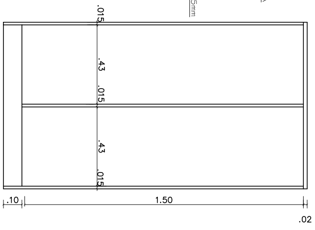
CORTE BB - ARMÁRIO
