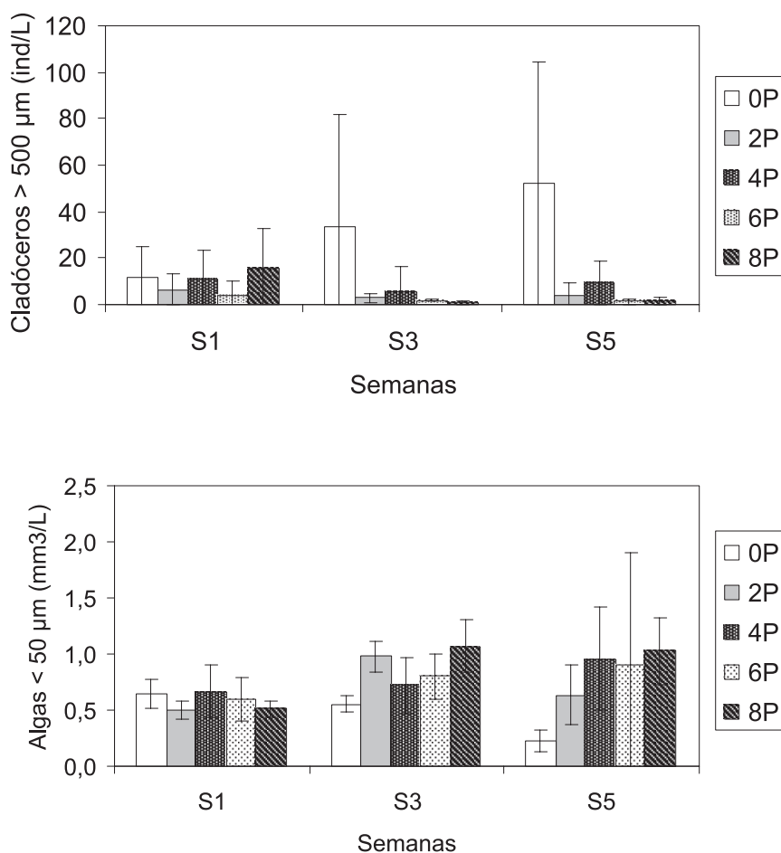
Figura 3. Média e desvio padrão das densidades de cladóceros grandes ( >500\ \mu\text{m} ) e do biovolume de algas pequenas (GALD <50\ \mu\text{m} ) nos cinco tratamentos (com 0, 2, 4, 6 e 8 peixes/mesocosmo) no início, meio e fim do experimento na ESEC Seridó.
