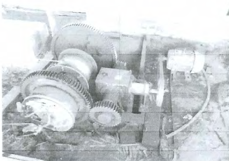
Fig. 3: Tambor do eixo do carrinho desprotegido.
