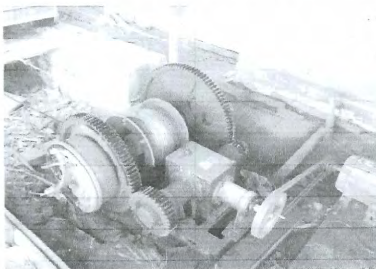
Fig. 4: Detalhe do tambor do eixo do carrinho desprotegido.
