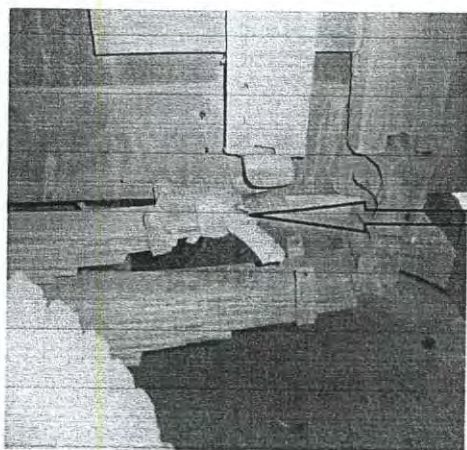
FEIXE DE MOLAS DA RODA TRASEIRA ESQUERDA PRESA COM LIGA DE BORRACHA
