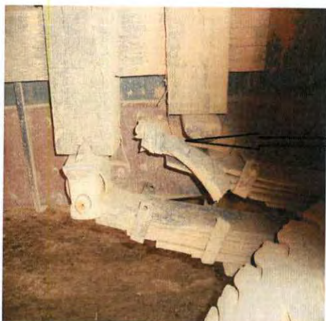
FEIXE DE MOLAS DA RODA TRASEIRA ESQUERDA PRESA COM LIGA DE BORRACHA
